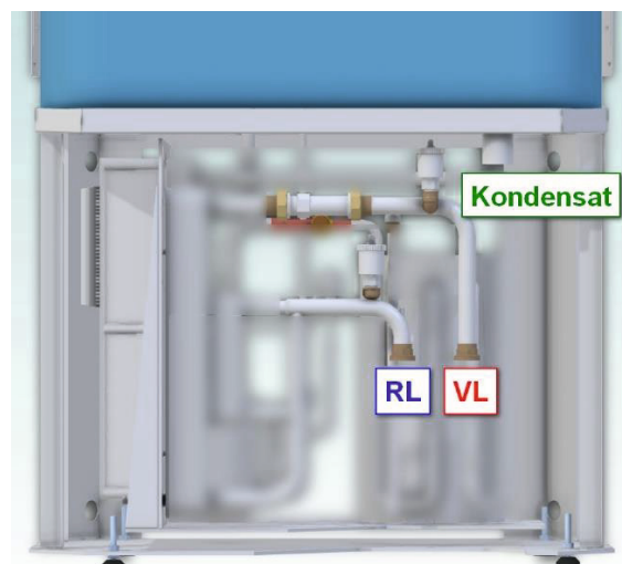
Abbildung 15: Hydraulik anschließen
