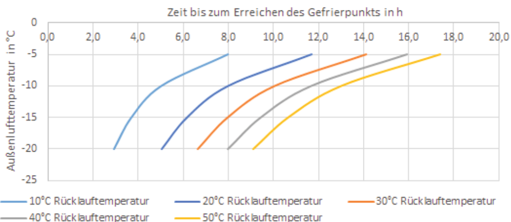
Abbildung 24: Zeitdauer bis zum Erreichen des Gefrierpunktes in den wasserführenden Bauteilen der Wärmepumpe
