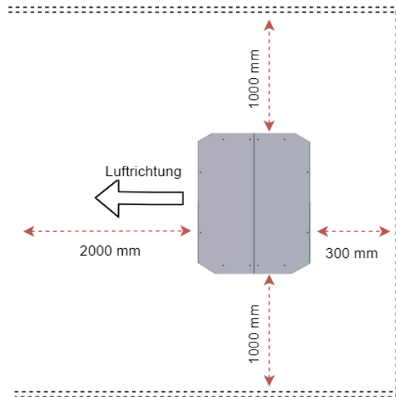
Abbildung 12: Mindestabstände
