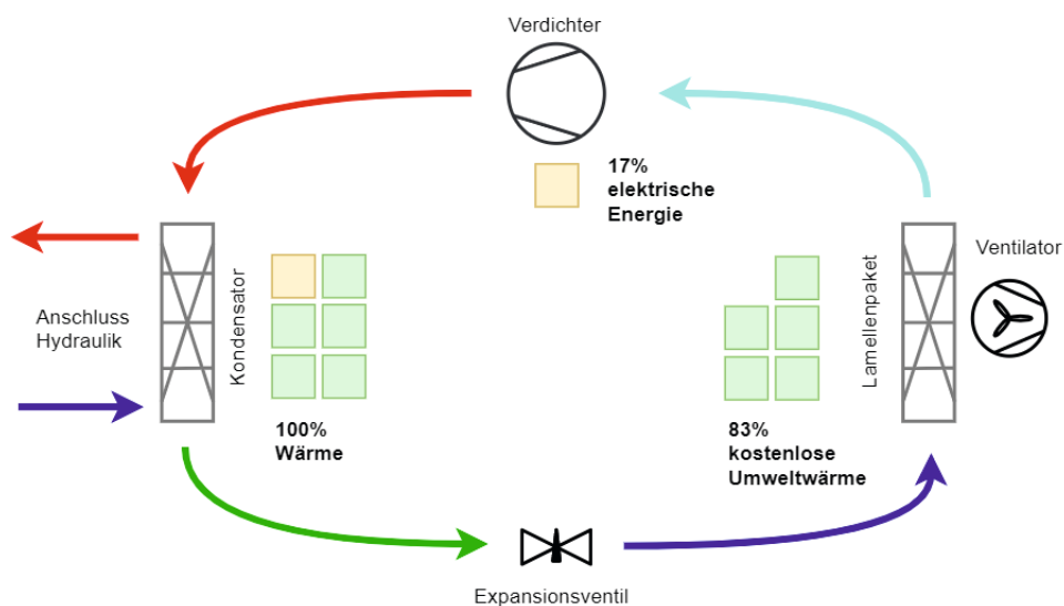
Abbildung 2: Funktionsprinzip
