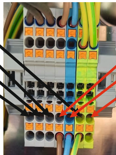
Abbildung 17: Elektrischer Anschluss Außeneinheit
