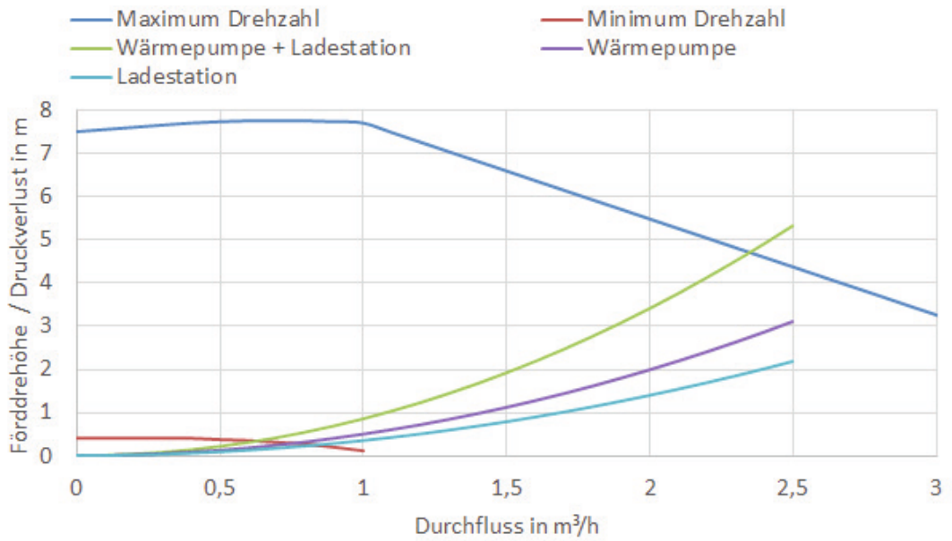
Abbildung 39: Pumpenkennlinie Grundfoss UPM3L 75/180 und Anlagenkennlinie
