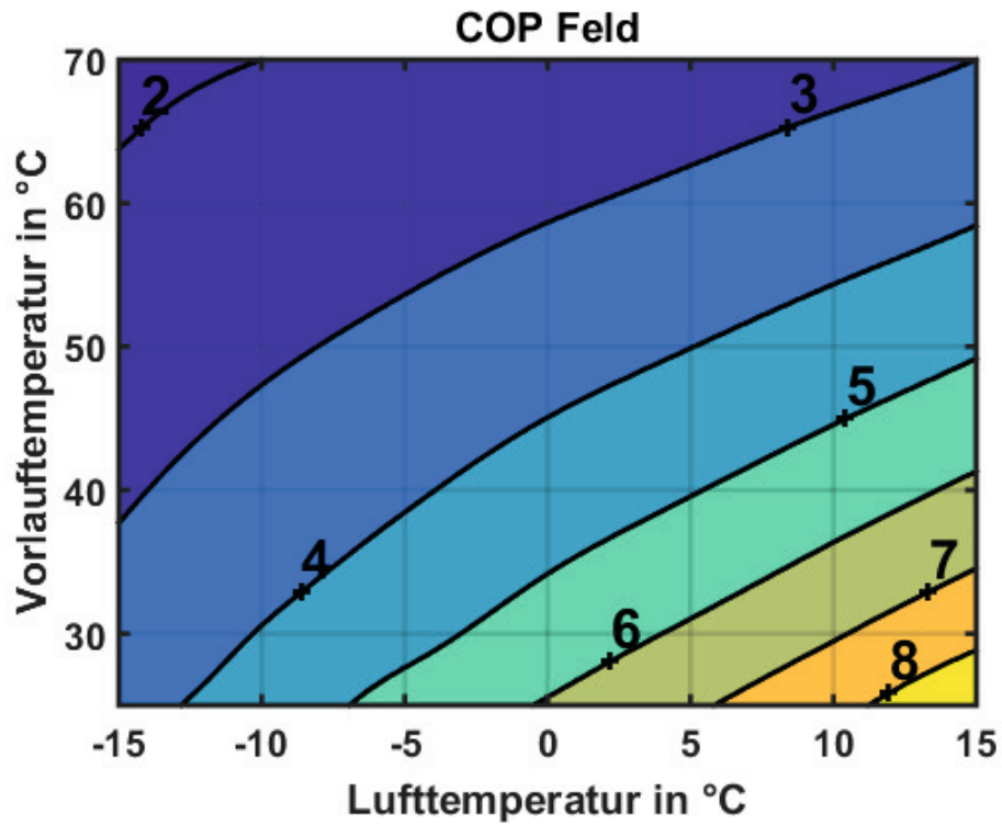
Abbildung 33: EU15L bei 11kW Heizleistung
