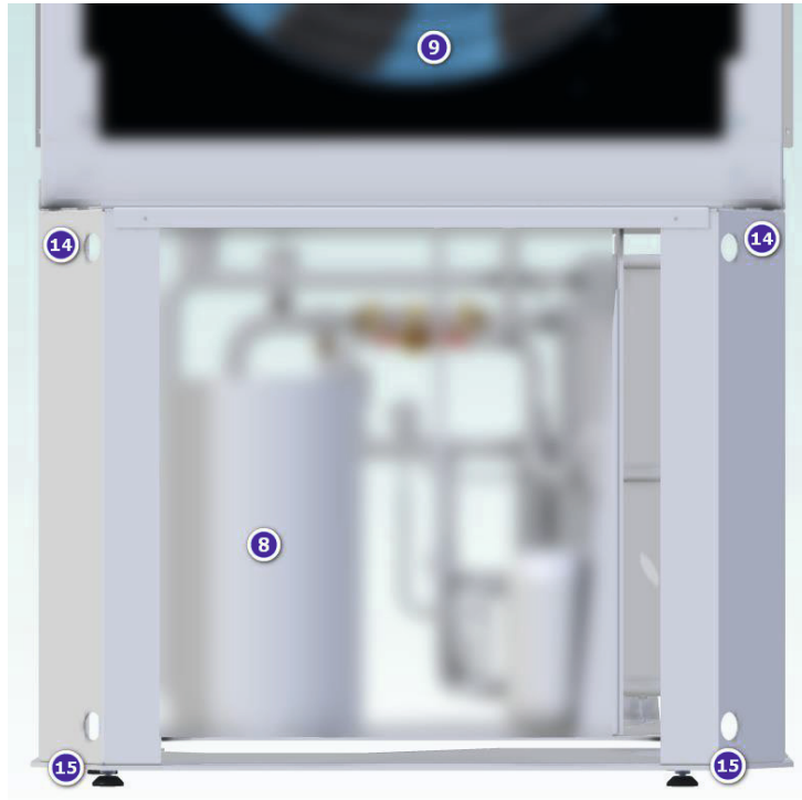
Abbildung 7: Ausstattung des Außengeräts: Ansicht hinten Kältekreis
