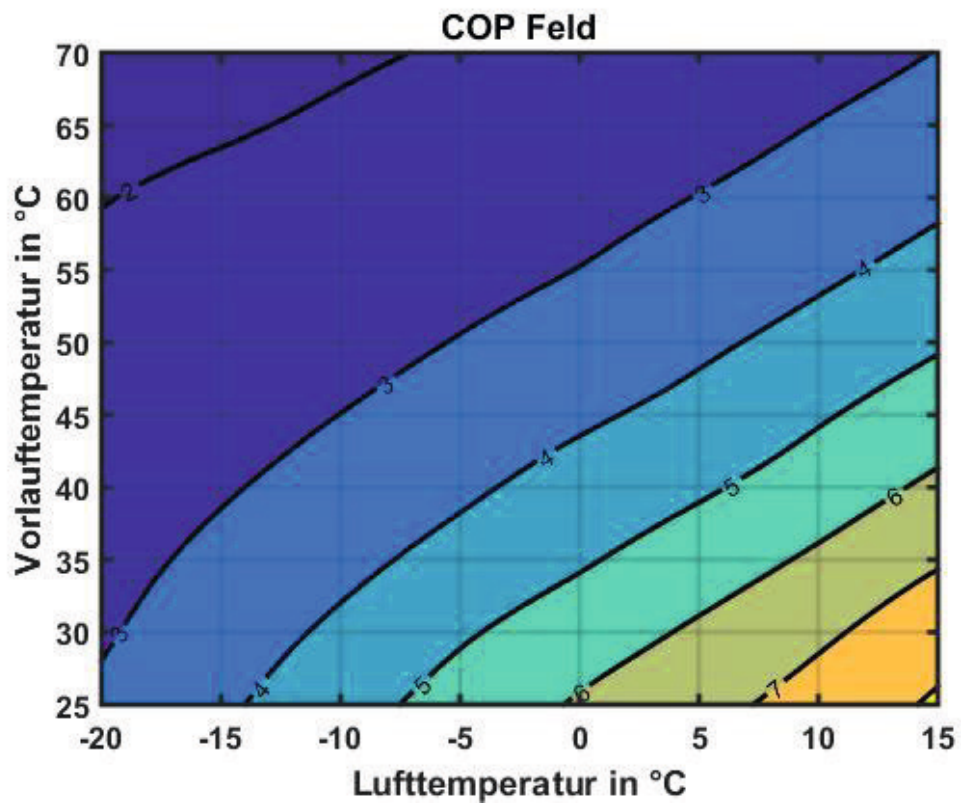
Abbildung 35: EU08L bei 6kW Heizleistung
