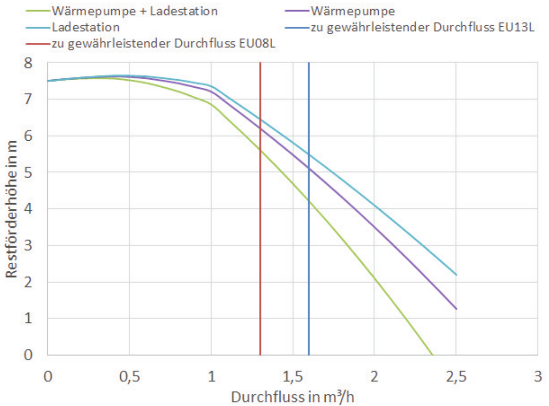
Abbildung 40: Restförderhöhe
