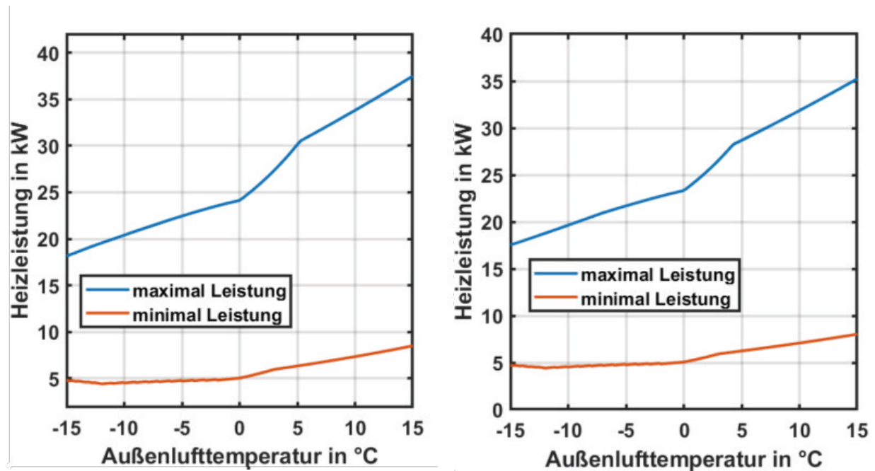
Abbildung 28: EU20L bei 5K Spreizung (links: 35°C Vorlauftemperatur / rechts: 55°C Vorlauftemperatur)
