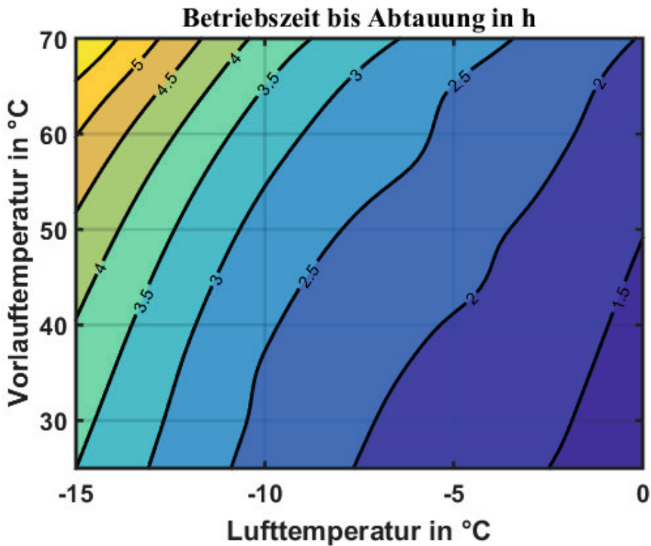
Abbildung 37: Betriebsdauer zwischen Abtauzyklen bei 9kW Heizleistung und 95% Luftfeuchte (EU13L)
